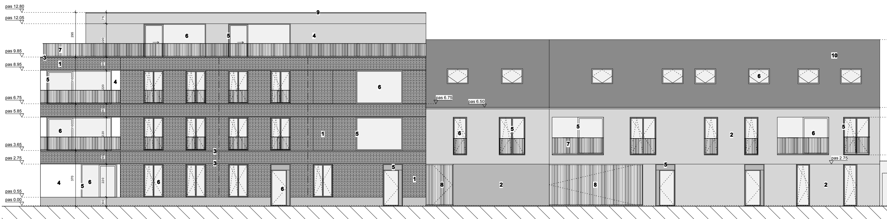
Voorgevel Vennestraat 1/150
